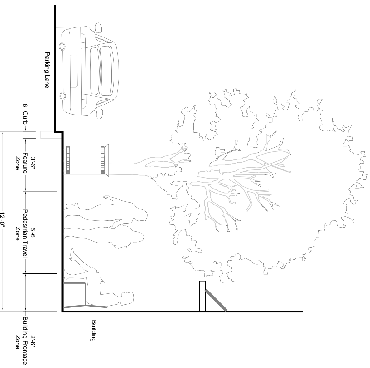
SECTION SCALE: 1/4" = 1'-0"
