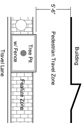
PLAN SCALE: 1/8" = 1'-0"
